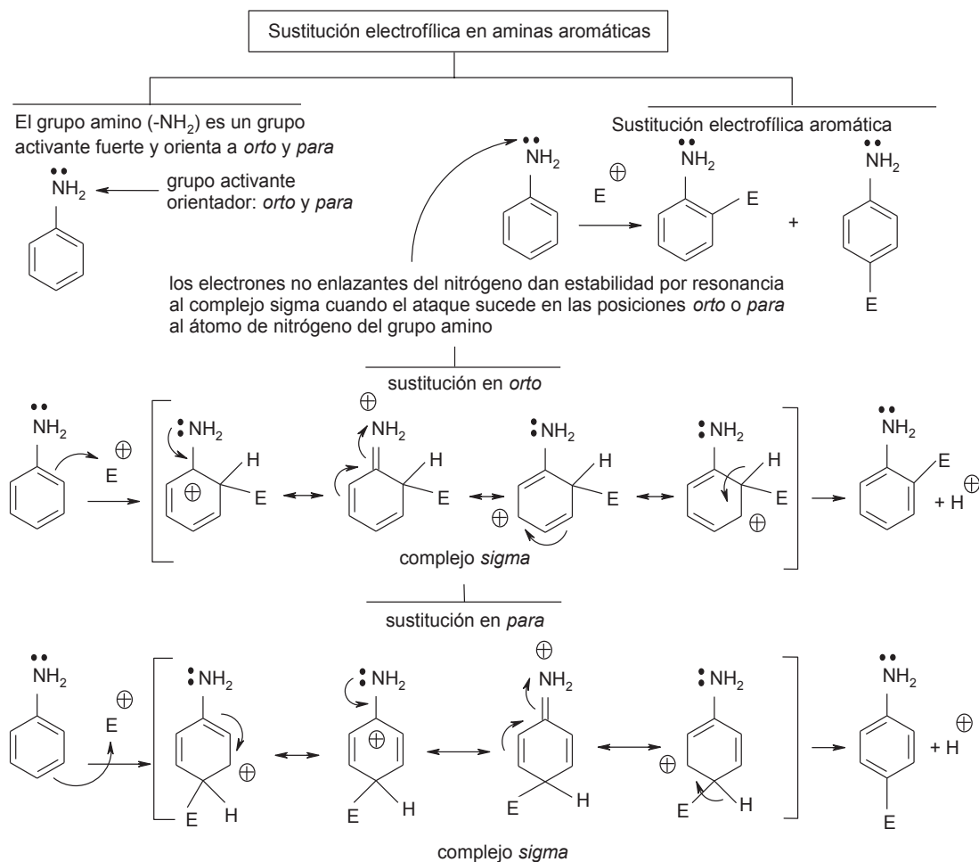
Esquema 2.7.1 Reacciones de sustitución electrofílica aromática
