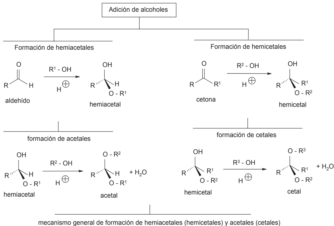
Etapa 1: formación del hemiacetal de un aldehído
