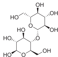
celobiososa (enlace glicosídico \beta -1, 4')
