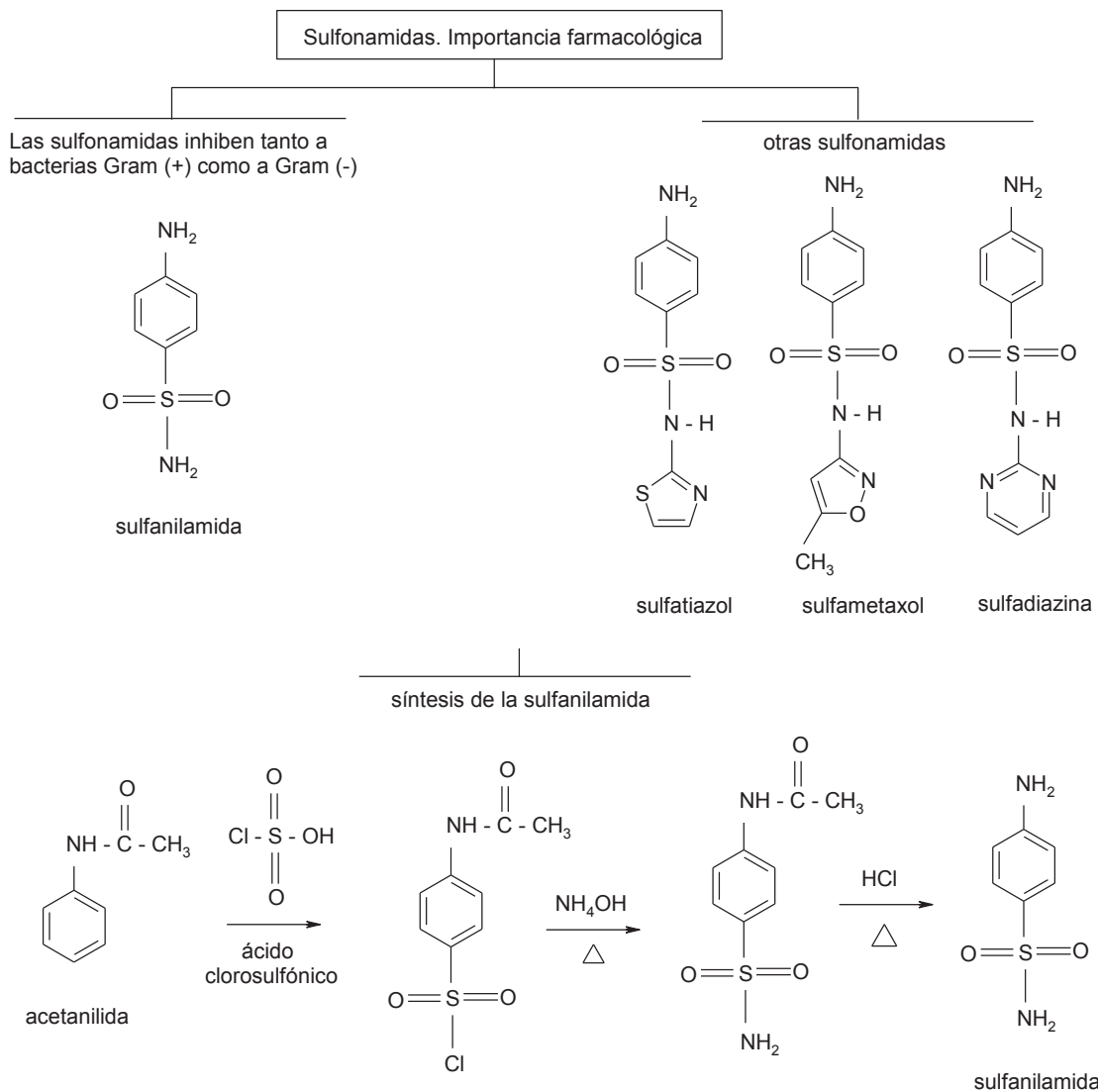
Esquema 2.9.1 Sulfonamidas
