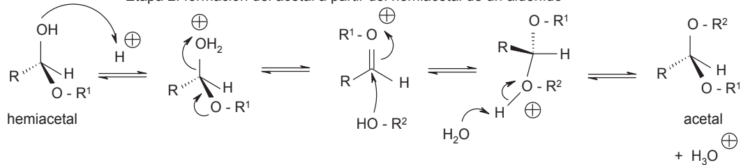
Etapa 2: formación del acetal a partir del hemiacetal de un aldehído
