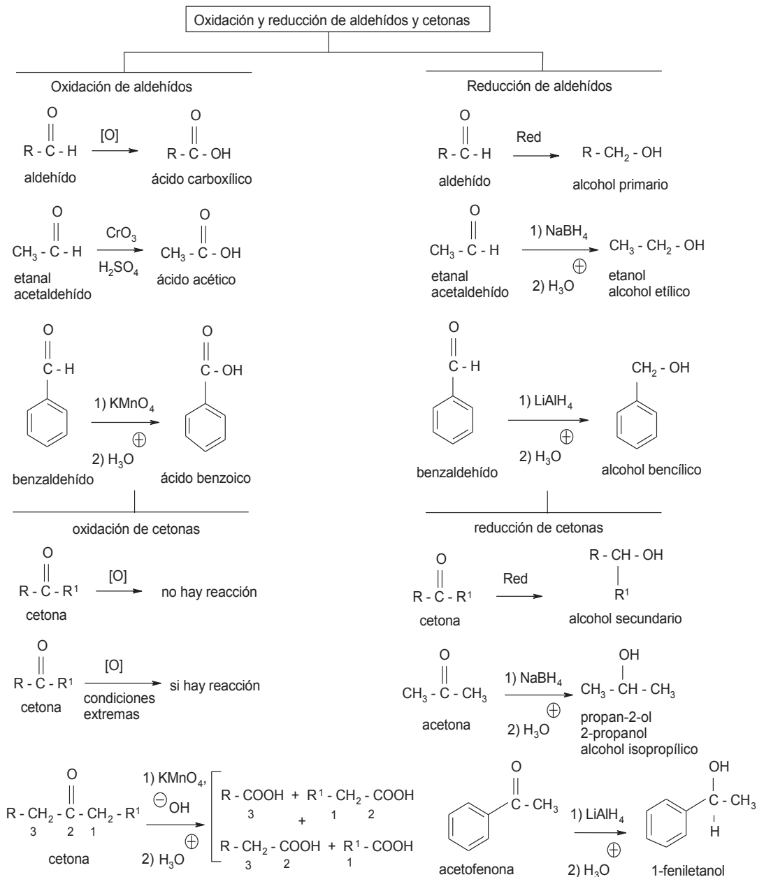
Esquema 3.14.1 Oxidación y reducción de aldehídos y cetonas
